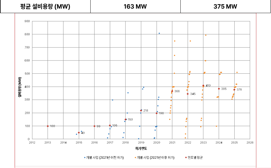
그림 8. 해상풍력 발전사업허가 설비용량 추이
