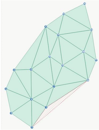
그림 7. 제주 한림 해상풍력단지의 터빈 배치와 들로네 삼각분할
