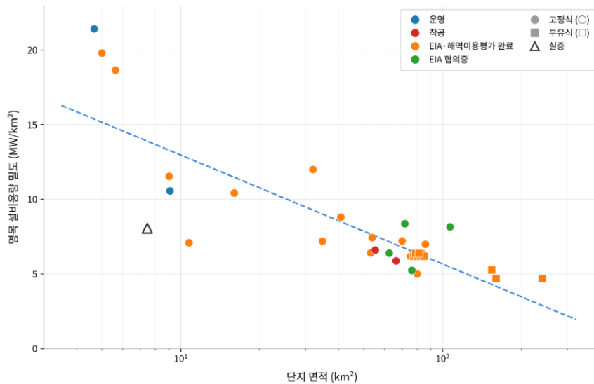
그림 4. 국내 해상풍력단지 면적과 설비용량 밀도의 관계
