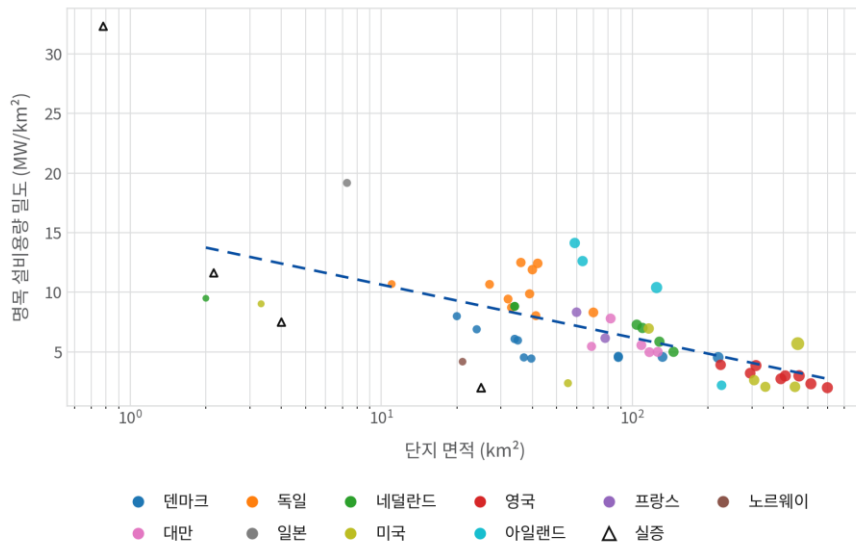
그림 1. 해외 해상풍력단지 면적과 설비용량 밀도의 관계
