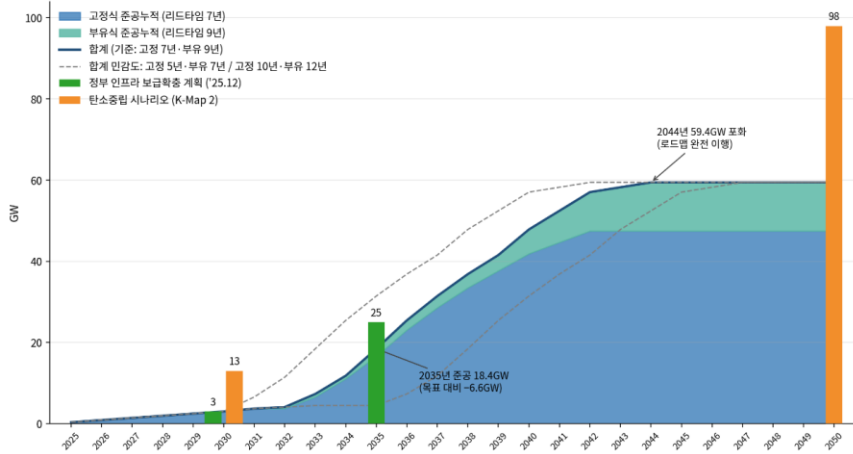
그림 3. 해상풍력 누적 보급 전망(2025~2050)
