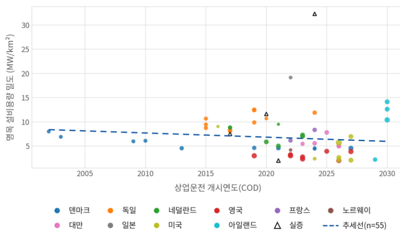
그림 2. 상업운전 개시연도별 해외 해상풍력 설비용량 밀도
