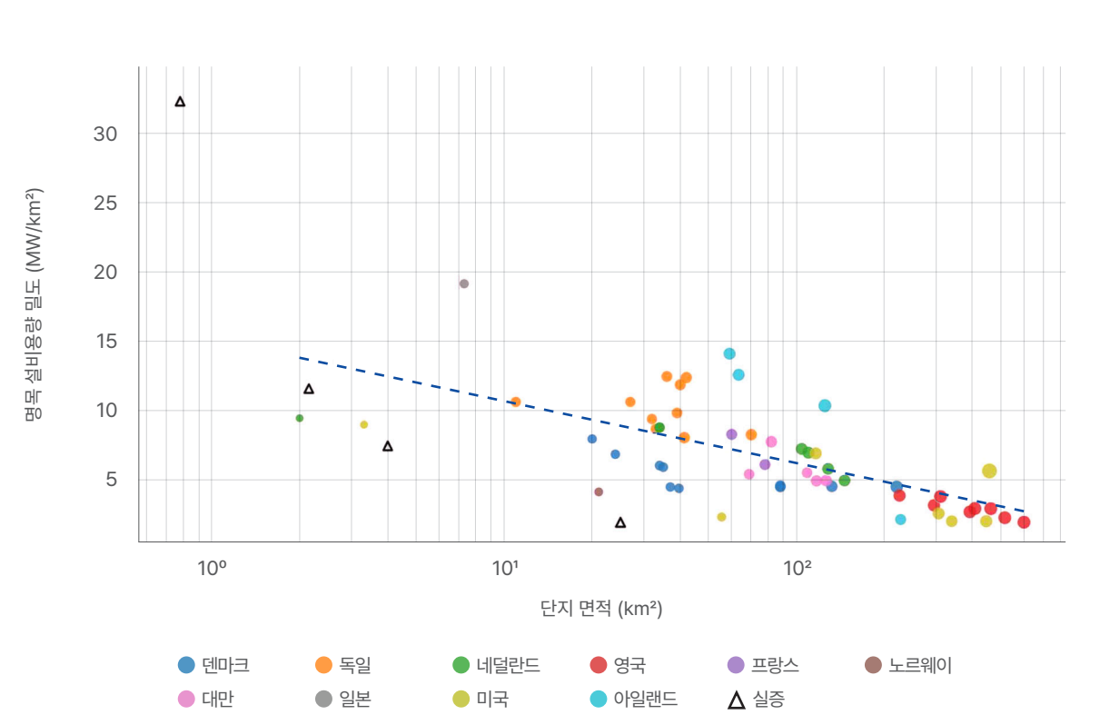
[그림 1] 해외 해상풍력단지 면적과 설비용량 밀도의 관계
