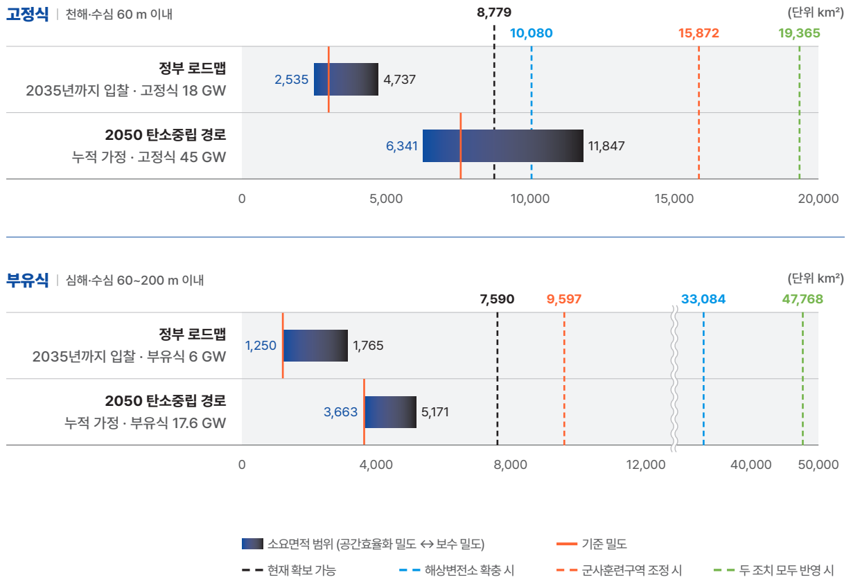
[그림 5] 기초형식별 발전지구 소요면적과 예비지구 가능해역 비교
